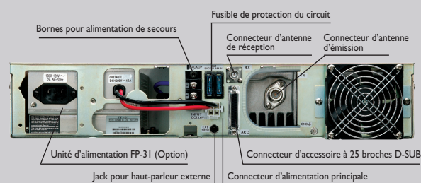
PANNEAU ARRIÈRE
