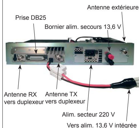
Face arrière série IF-FR5100D 220V
